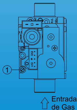
Válvula de gas Sit
